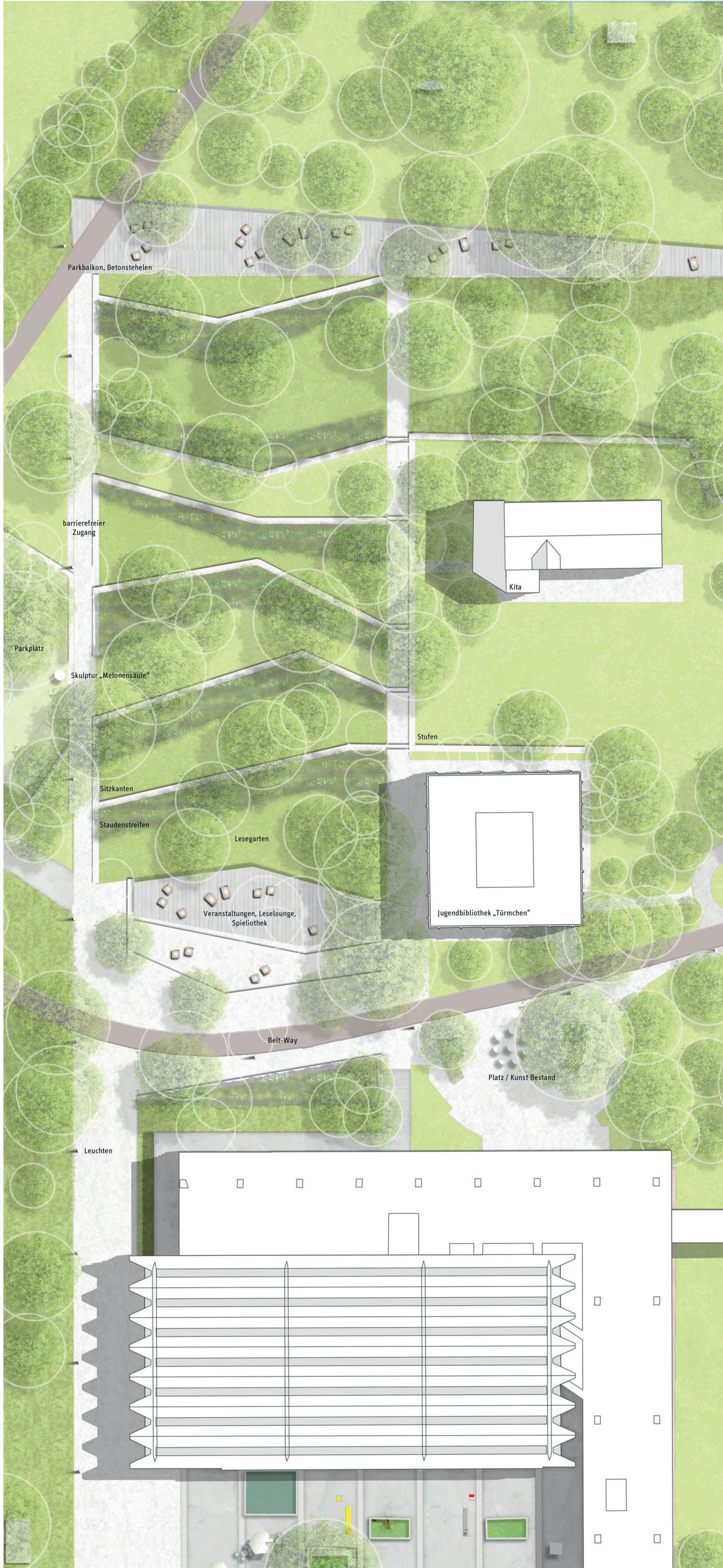
Rathausgarten M 1 : 250
