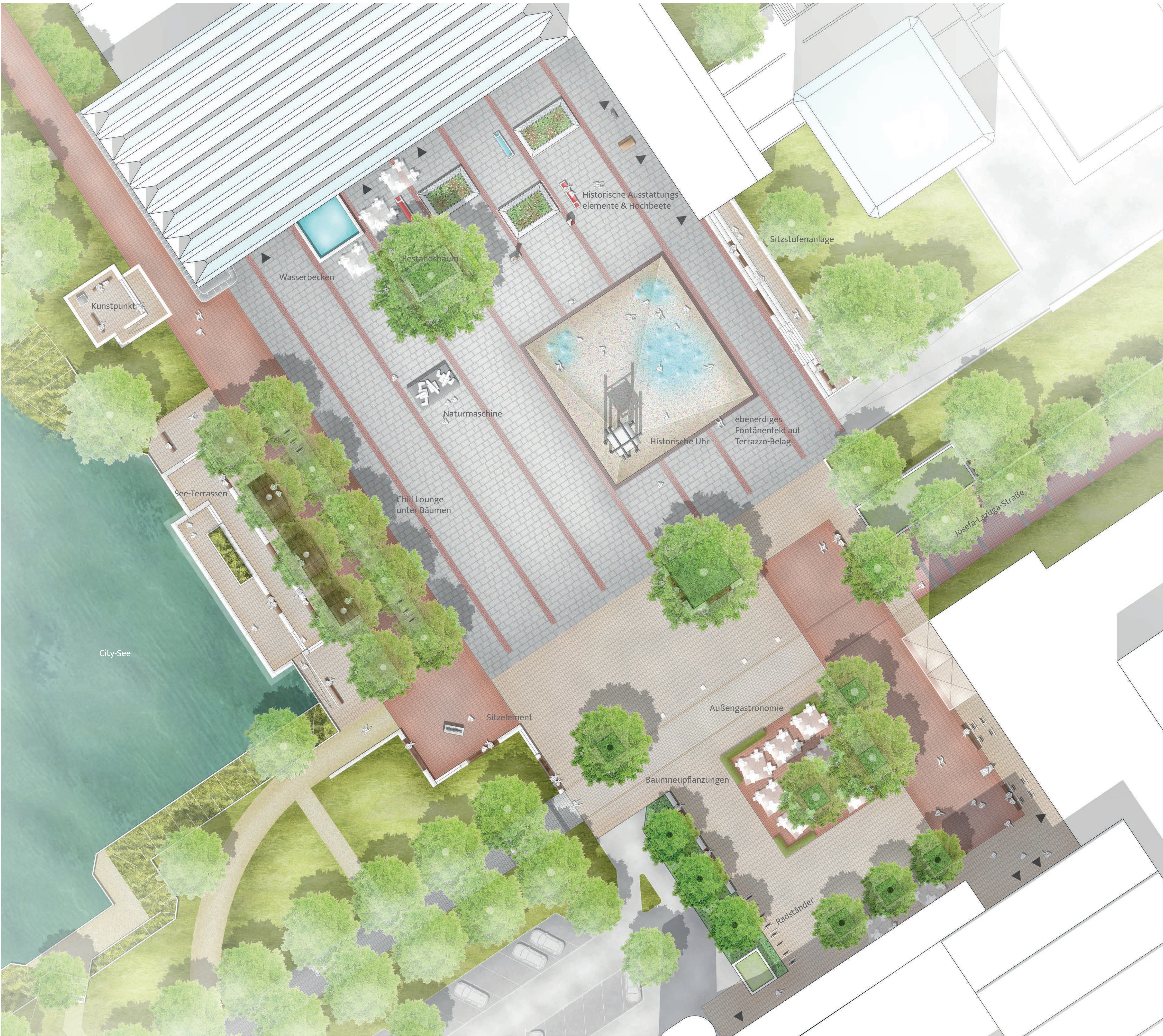
Bereich Creiler Platz M 1:250
